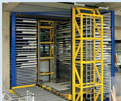
Vollautomatisches Blechlager
